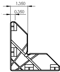
CD-H1AR Storm Door Corner
